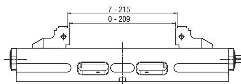
Doppio Bloccaggio
