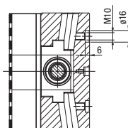
SEZIONE C-C
