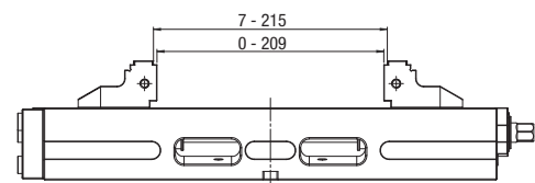
Fissa
