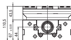
SEZIONE C-C
