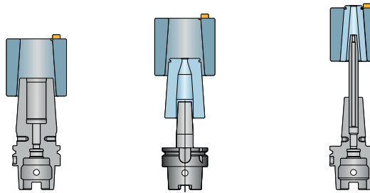
Campana di raffreddamento per mandrini a calettamento a norme DIN
